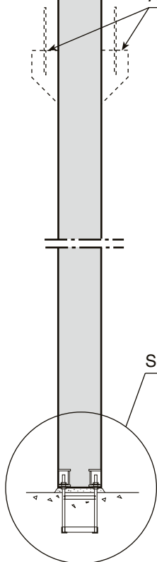
SEKTION GENOM PELARE OCH FACKVERK
