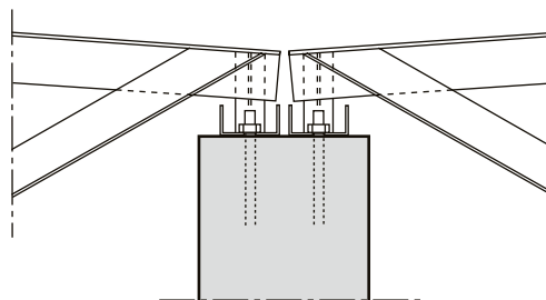
DETALJ 1 DUBBELT FACKVERKSUPPLAG
