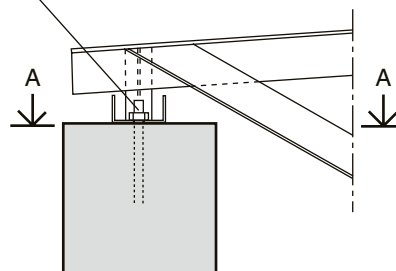
DETALJ 1 ENKELT FACKVERKSUPPLAG
